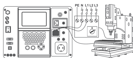
Test impedancie slučky
